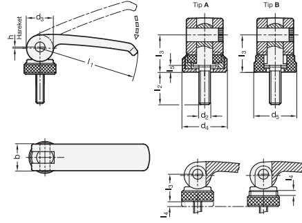
GN 927.5-B-Điřli saplamalı, ayar somunu olmayan plastik temas plakası
