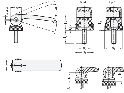
GN 927.5-A- Dişli saplamalı, ayar somunlu plastik temas plakası
